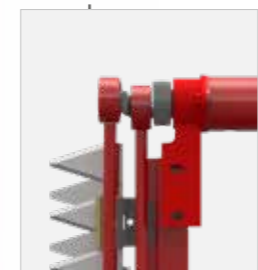
Drehelastische Kupplung Torsionally flexible coupling
